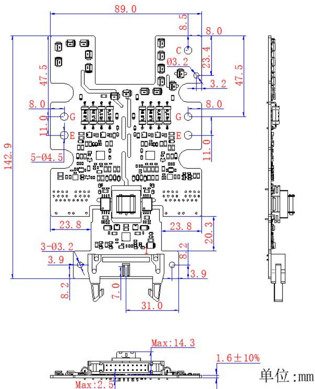
图4 3D及机械尺寸图
