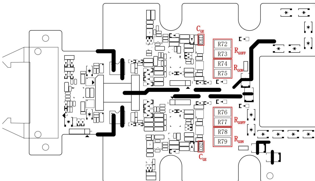
图 3a 门极电阻电容位置指示图（贴片电阻）
