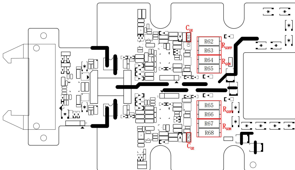
图 3b 门极电阻电容位置指示图（直插电阻）
