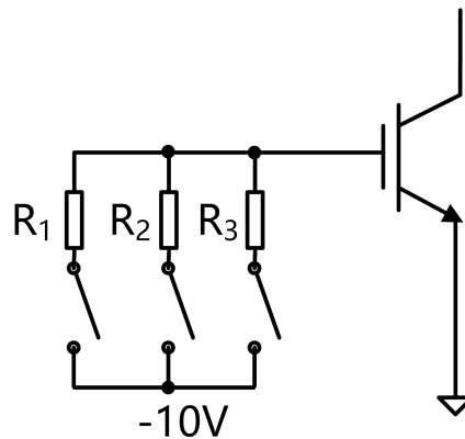
图 11 分级关断原理图
