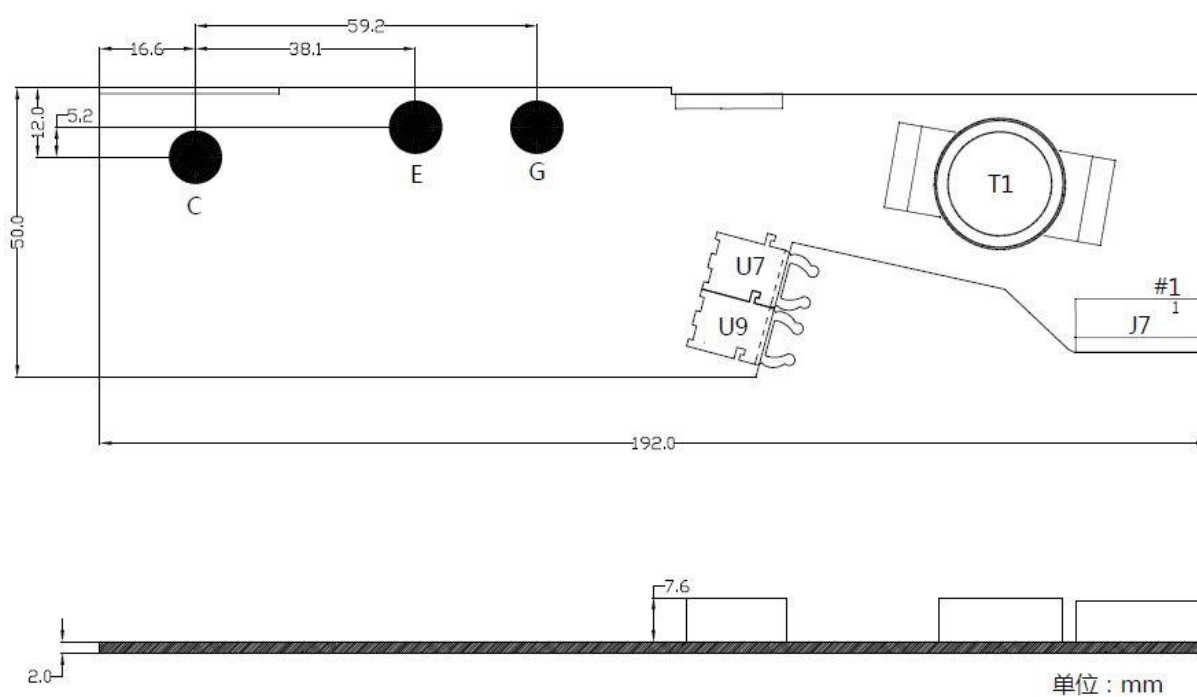
图 4 1FSD08110-V 尺寸图
