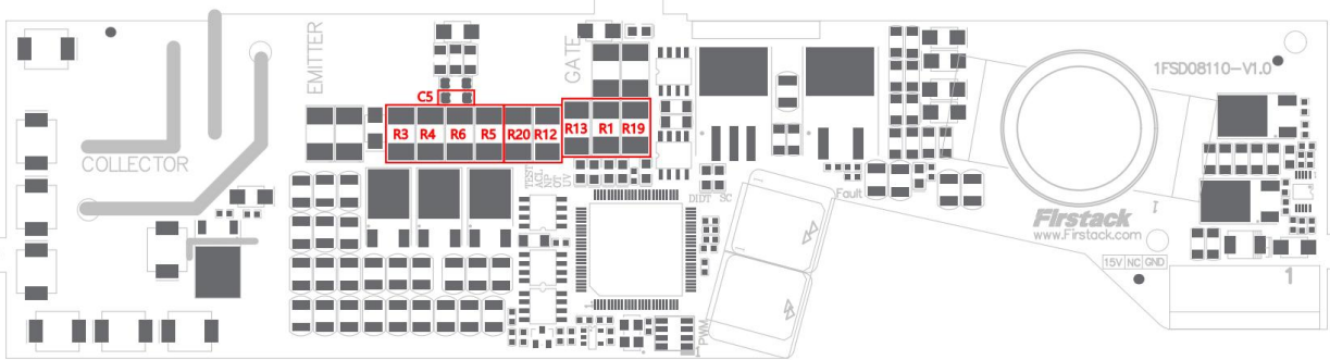
图 17 门极电阻位置指示图
