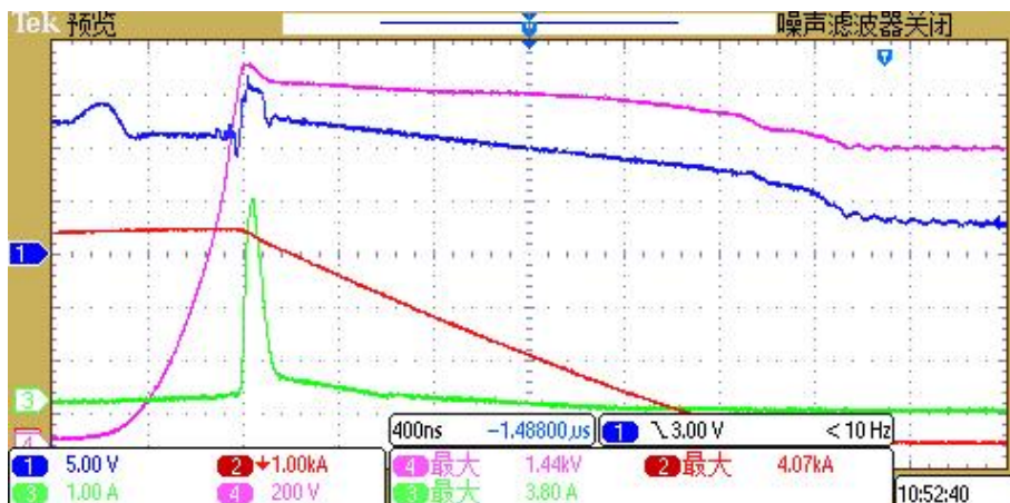
图 10 数控有源钳位波形
