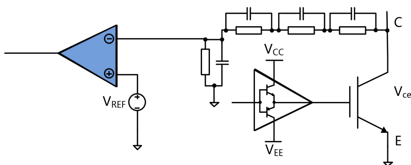
图 7 V_{CE} 退饱和检测电路
