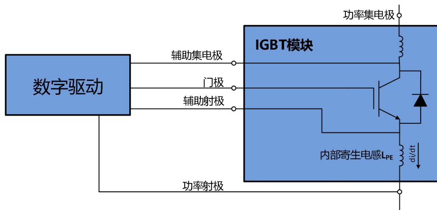
图 6 di/dt 检测电路
