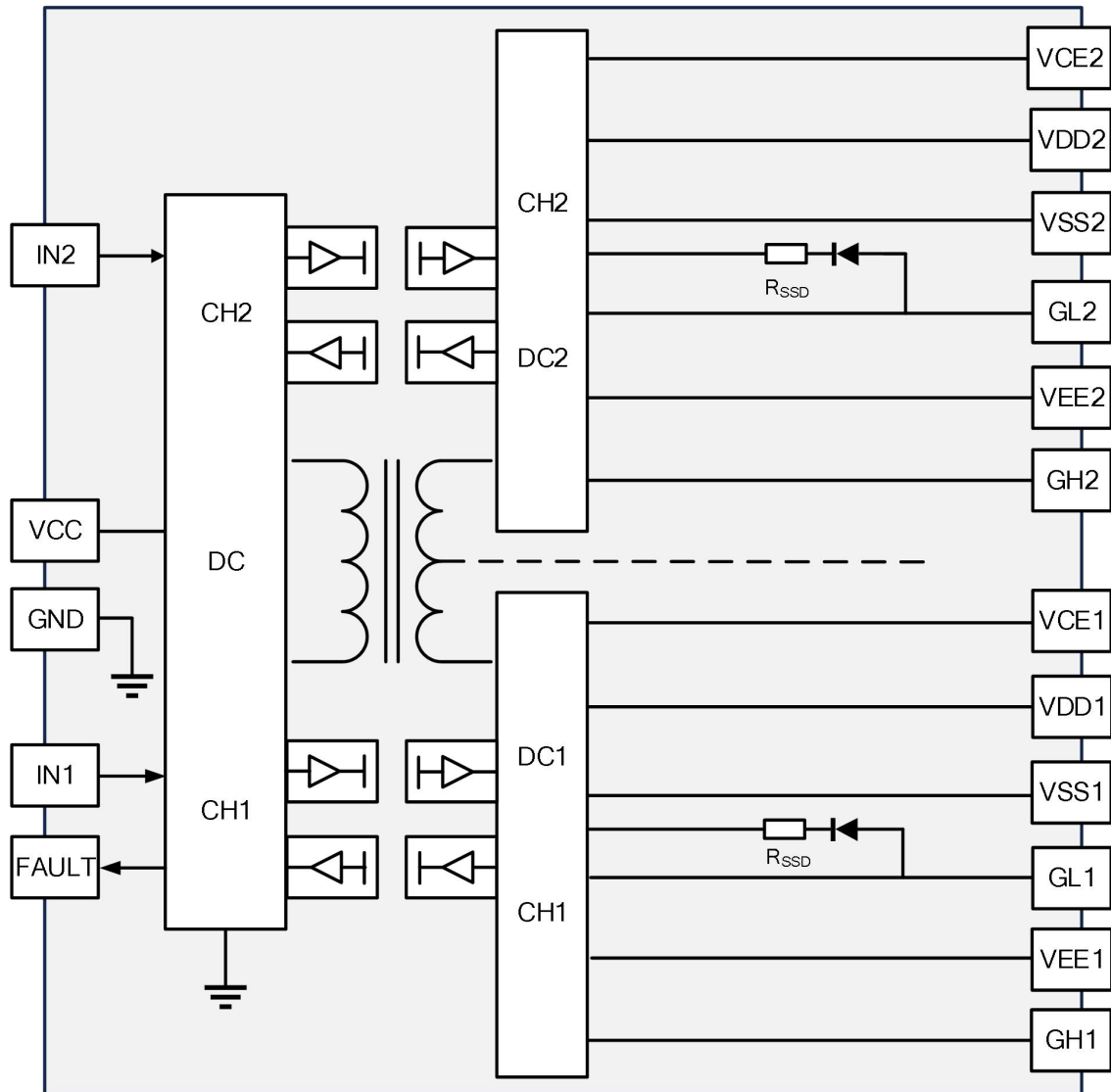
图 2 功能框架图
