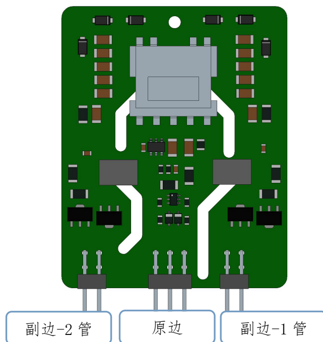
图 5 2FSC0110T12D1 驱动板原副边示意图
