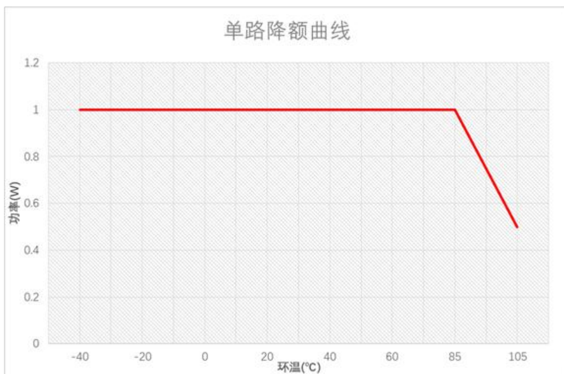
图 4 降额曲线图
