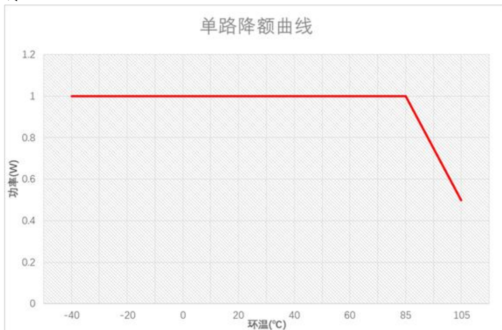
图 4 降额曲线图
