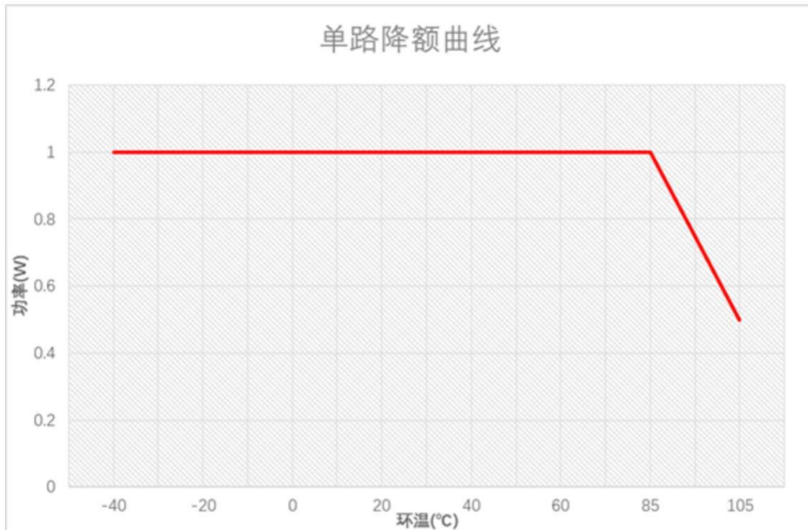
图 4 降额曲线图
