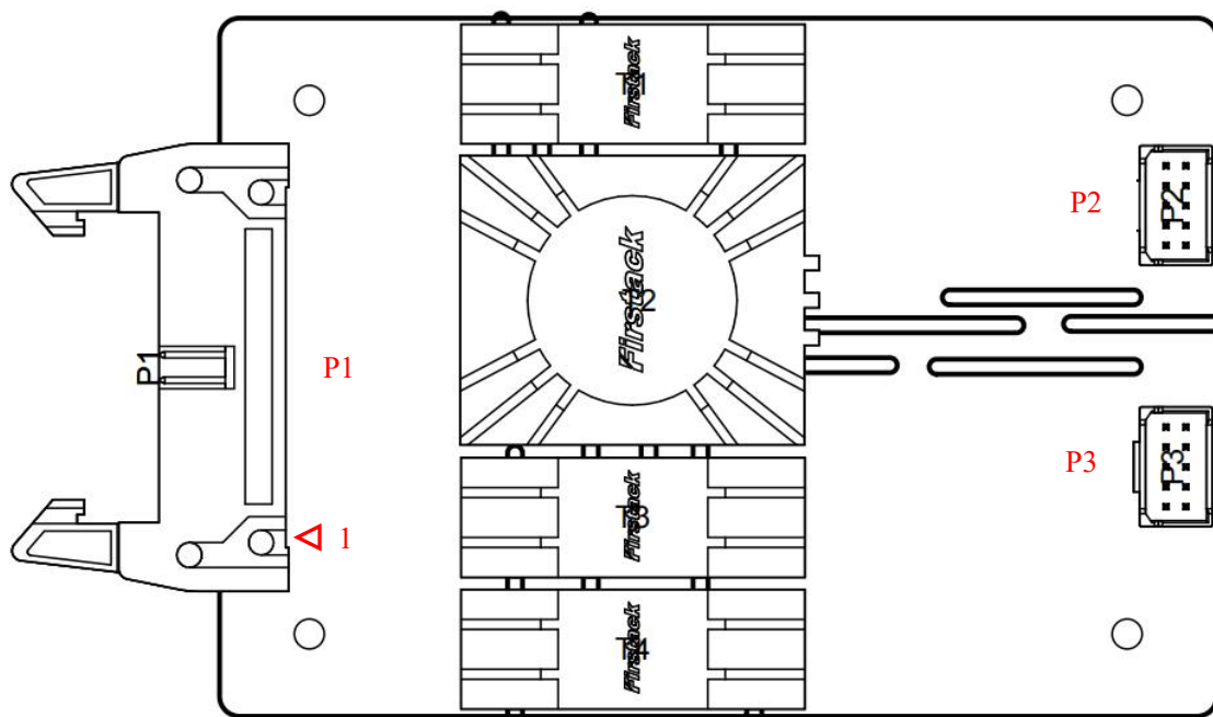
图 3 接口定义图
