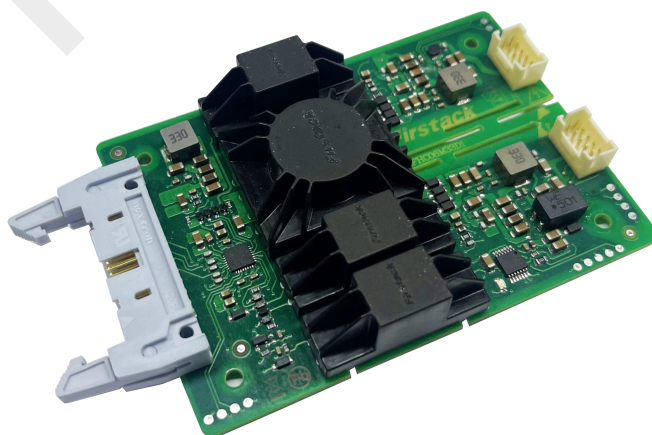
图 1 2FHC06M33XX
