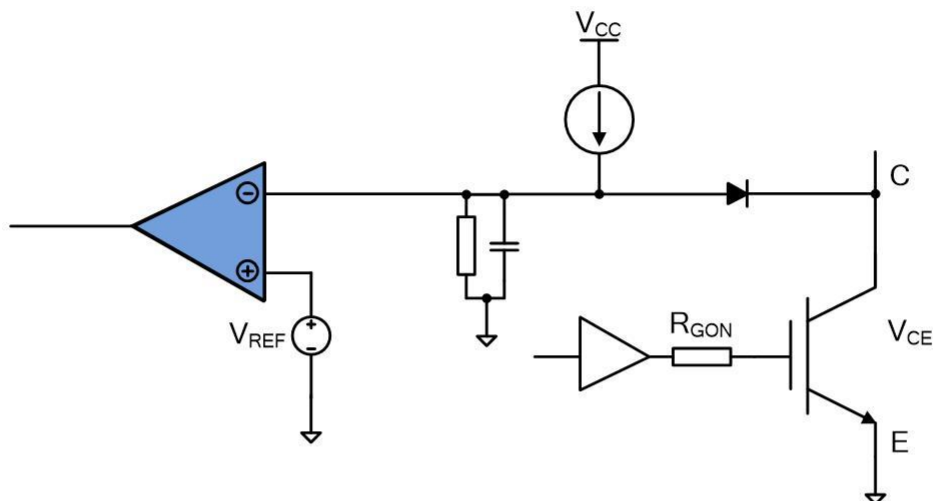
图 4 V_{CE} 退饱和检测电路
