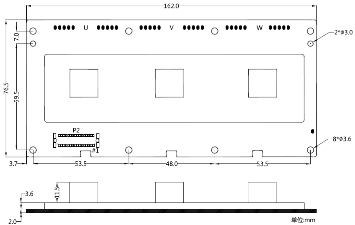
图 3 尺寸图
