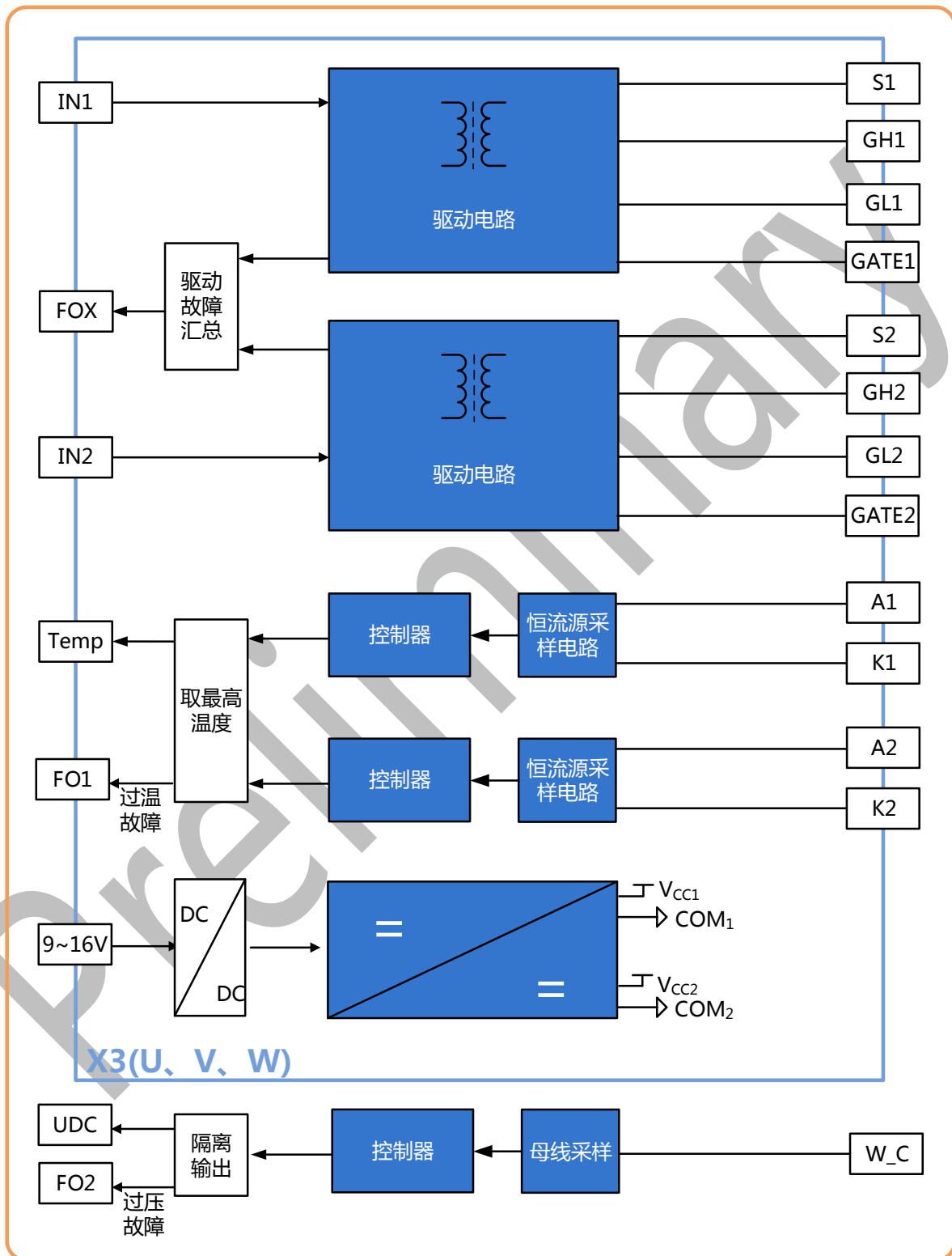
图 2 系统框架图
