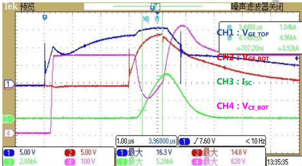
图 5 6MBI800XV-075V-01 在 450V 下的短路波形
