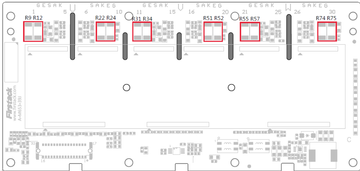
图 8 门极电阻位置指示图
